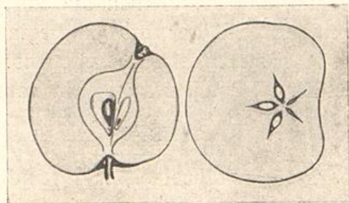
Abb. 13. Längs- und Querschnitt durch einen ungleich entwickelten Apfel. Die größere Hälfte enthält größere und zahlreichere Samenerne. Nach Molisch.
