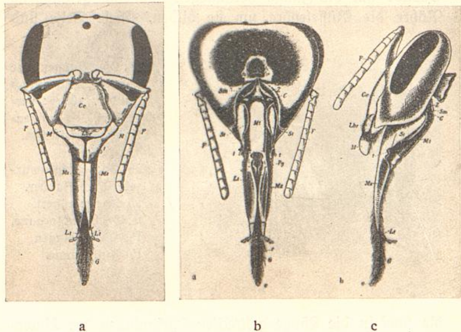
Abb. 3. Kopf und Mundteile einer Arbeiterin: a von vorne, b von hinten, c von der Seite. Nach Zander. 8 \times vergrößert.
