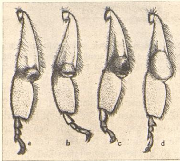
Abb. 7. Das Anwachsen des Vollenballens durch Nachschieben von unten und Heraufschieben auf dem glatten Boden des Rörbchens. Aus v. Buttel-Reepen nach Gasteel.
