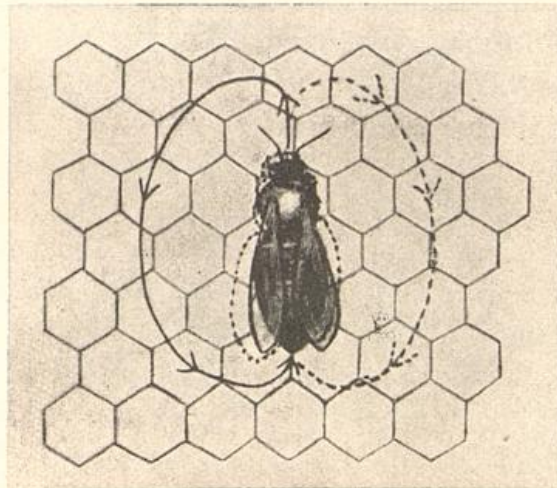
Abb. 11. Schwänzeltanz einer Biene, die von reicher Pollentracht heimgekehrt ist. Die Pfeile geben die Richtung der Bewegung an, die unter schnellem Hin- und Herschwänzeln des Hinterleibs bald nach rechts, bald nach links ausgeführt wird. Nach v. Frisch.
