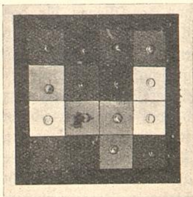
Abb. 8. Nachweis des Farbensinns. Ein blaues Blatt in der Grauerie; alle Papiere mit einer Glasplatte überdeckt; darauf reine leere Uherschälchen. Die auf Blau dressierten Bienen versammeln sich über dem blauen Papier, obwohl auch dieses Schälchen kein Futter enthält. Nach v. Frisch.
