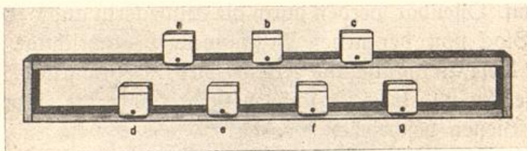
Abb. 9. Anordnung der Duftkästchen zur Duftdressur. Nach v. Frisch.
