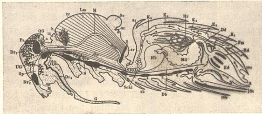
Abb. 4. Schematischer mittlerer Längsschnitt durch eine Arbeitsbiene.
