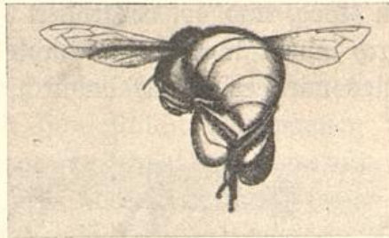
Abb. 6. Arbeitsbiene mit Höschen, während sie mit dem Pollenkamm des rechten Hinterbeins den Blütenstaub aus der Bürste des linken Hinterbeins herauskämmt. Aus v. Buttel-Reepen nach Gasteel.
