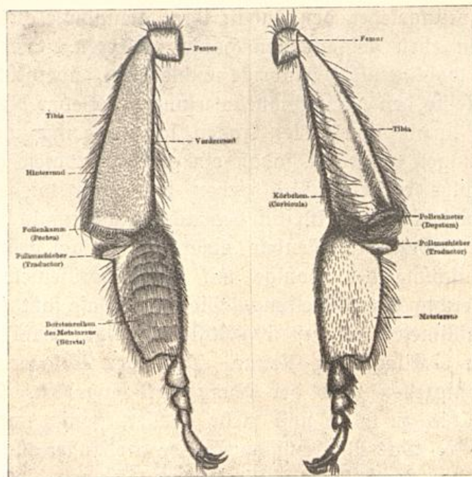
Abb. 5. Linkes Hinterbein einer Arbeitsbiene, links von innen, rechts von außen. Aus v. Buttel-Reepen nach Gasteel.
