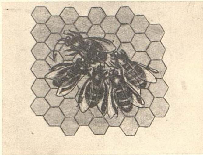
Abb. 10. Rundtanz einer Biene, die von reicher Nektartracht heimgekehrt ist. Der Pfeil gibt die Richtung der Bewegung an. Nach v. Frisch.
